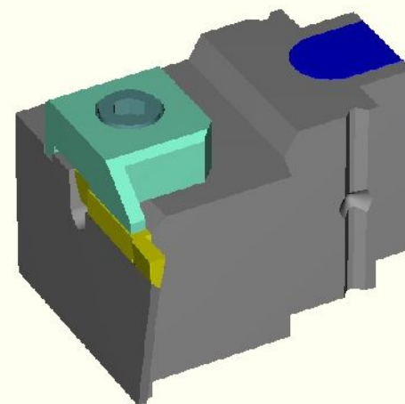
特殊溝入れホルダー-BTS
